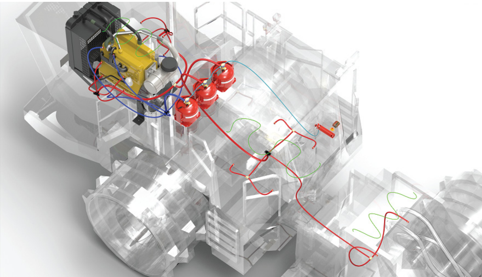
Sistema Automático de Detecção e Combate a Incêndio Veicular de Agente Duplo.
