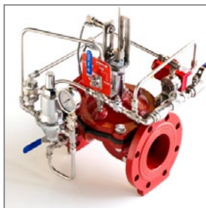
Válvulas Hidráulicas
